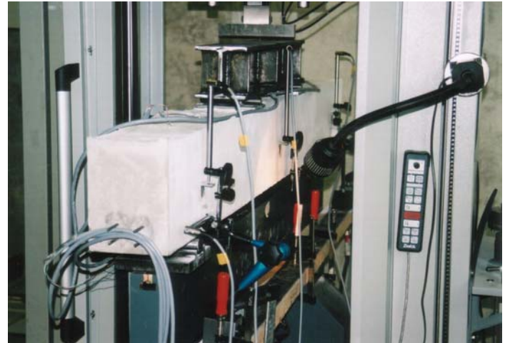
Versuchsaufbau
