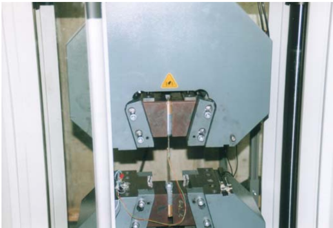
Prüfung Spannstahl
