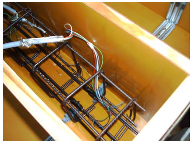
Applizierte DMS am Spannstahl
