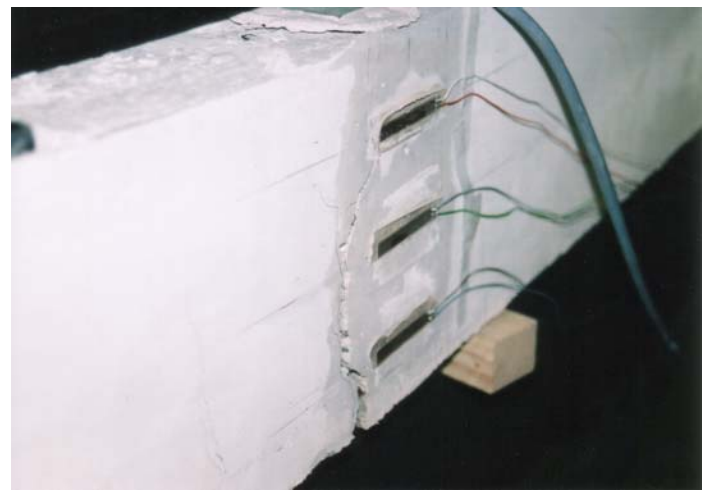
Versagen
