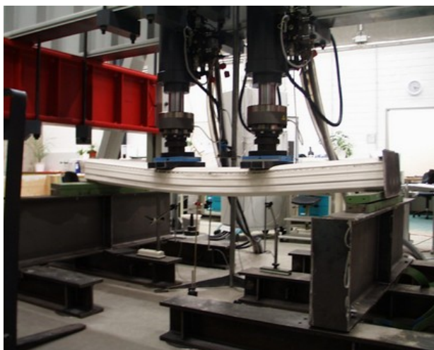
Biegezugversuch
