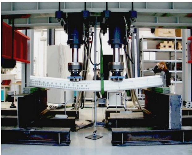
Biegezugversuch
