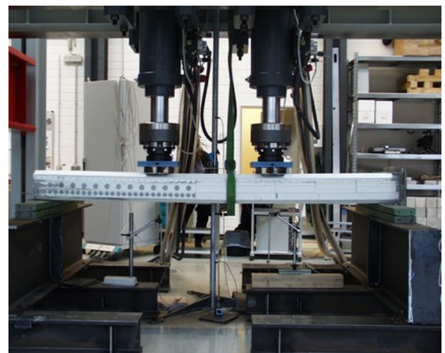
Biegezugversuch
