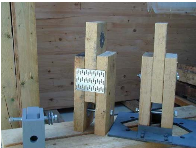
Versuchskörper Nagelplatte Einpreßdübel
