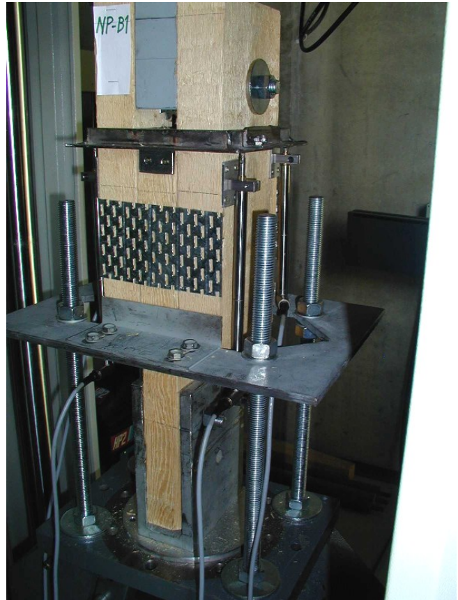
Versuchsaufbau – Prüfung in der Z400E
